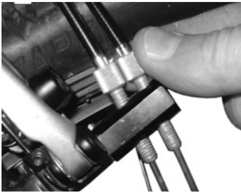
Afbeelding 154: Bij Rohloff naafversies met interne schakelaansturing zit de kabelafsteller op de tegenhouder van de kabel.
