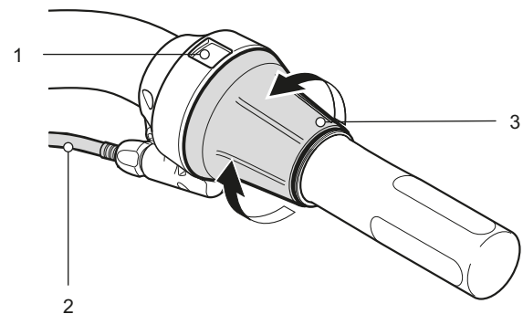
Afbeelding 49: Versnelling SHIMANO SL-C30000-7O
